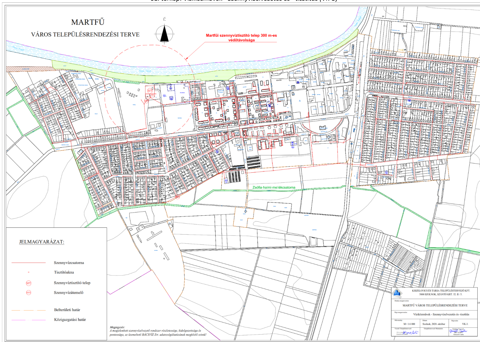
61. térkép: Víziközművek - Szennyvízelvezetés és -tisztítás (VK-3)
